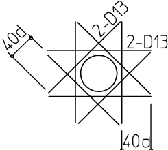
開口部補強筋
