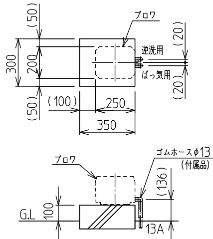
プロフ据付図(例)(尺度 N.T.S)
