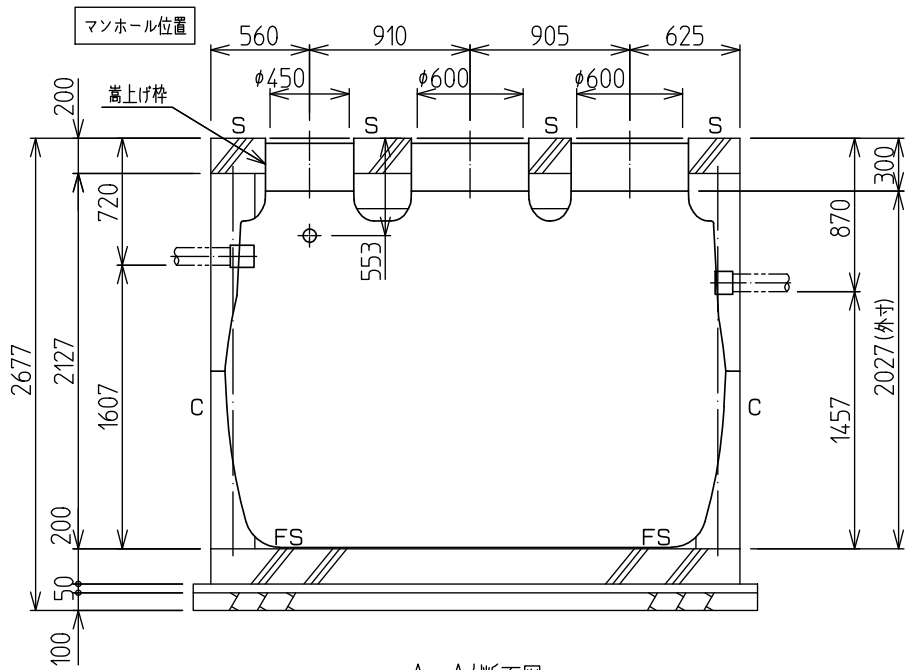
A-A'断面図
