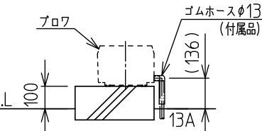
フロウ据付図(例)(尺度 N.T.S.)
