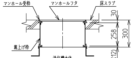
丸型マンホール枠詳細図(例) (尺度 N.T.S.) (嵩上げ枠AJW型を使用した場合)
