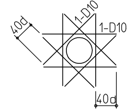
開口部補強筋
