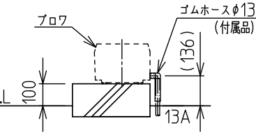
フロワ据付図(例)(尺度 N.T.S)
