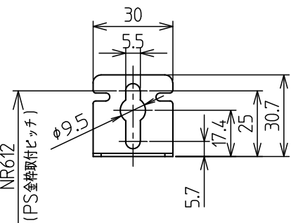
■C部詳細図(尺度1/2)
