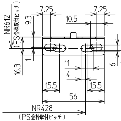
■D部詳細図(尺度1/2)
