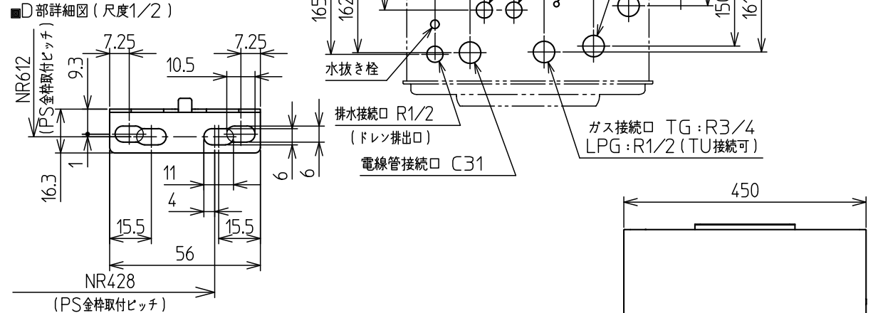
■D部詳細図(尺度1/2)
