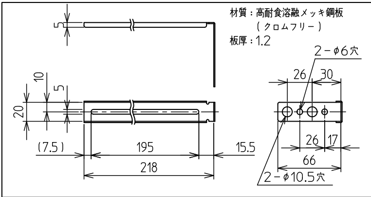
■本体取付板（付属部品）（尺度フリー）
