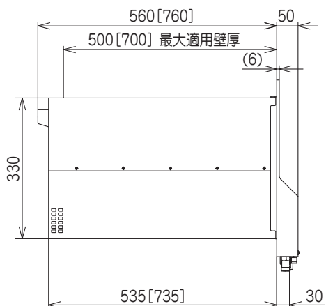
〈WF-S1602AT/ATL の場合〉
