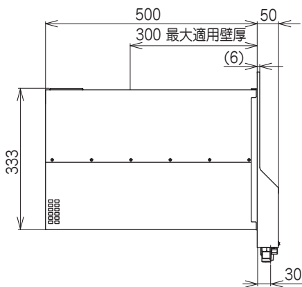
〈WF-S1602AT-C の場合〉
