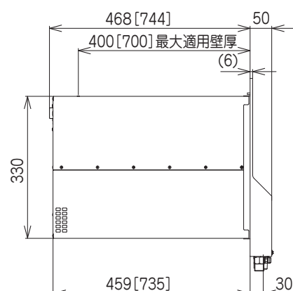
〈WF-807AT/ATL の場合〉
