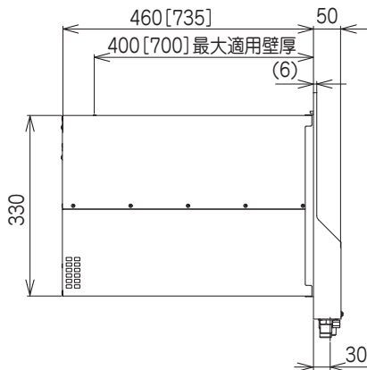
〈WF-1613AT/ATL の場合〉
